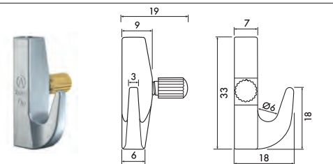
9.4219 7 kg
